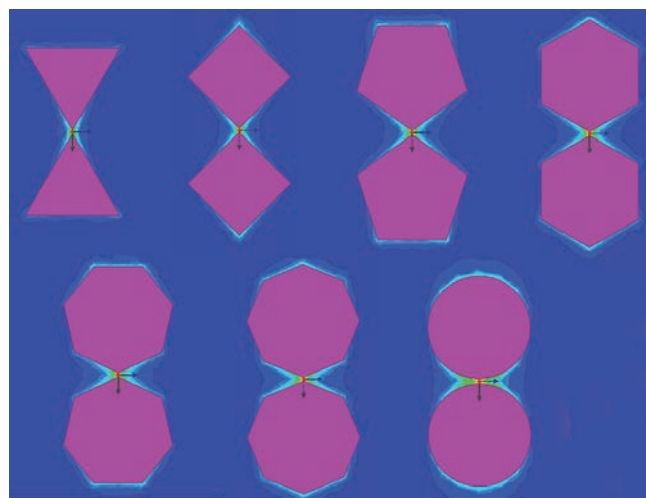
شکل ۲ | ساختار نانوآنتن‌ها
